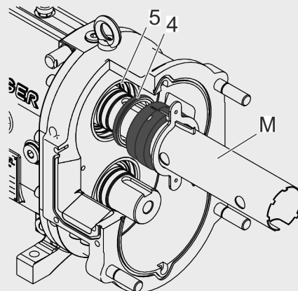
Supports du grain fixe - monter les faces de frottement
