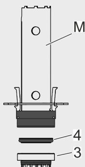
Supports du grain tournant - monter les faces de frottement
