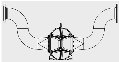
Modèle col de cygne
