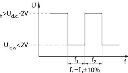
Ausgangssignal Output signal
